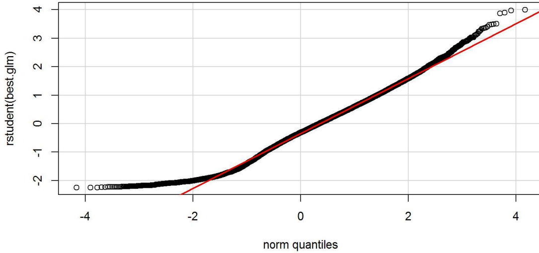
Negative Binomial Fit, WAG 1995/96-2004/05
