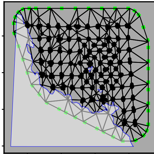
CT 20km
